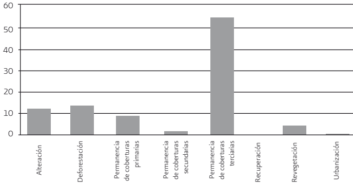
Figura 28. Procesos de cambio del municipio de Peribán, 1976 a 2000 (porcentajes)
